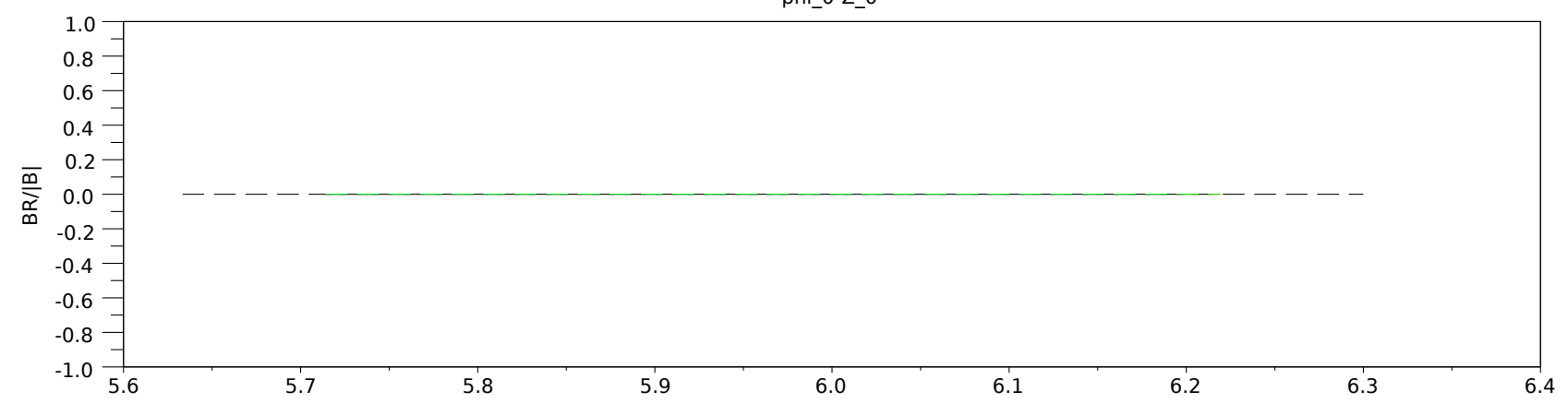
phi_0-Z_0
